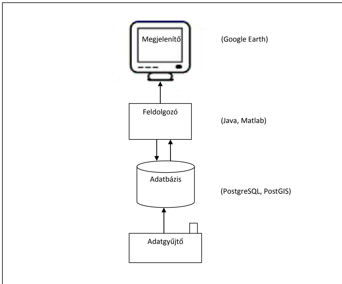
9. ábra – Architektúra diagram
